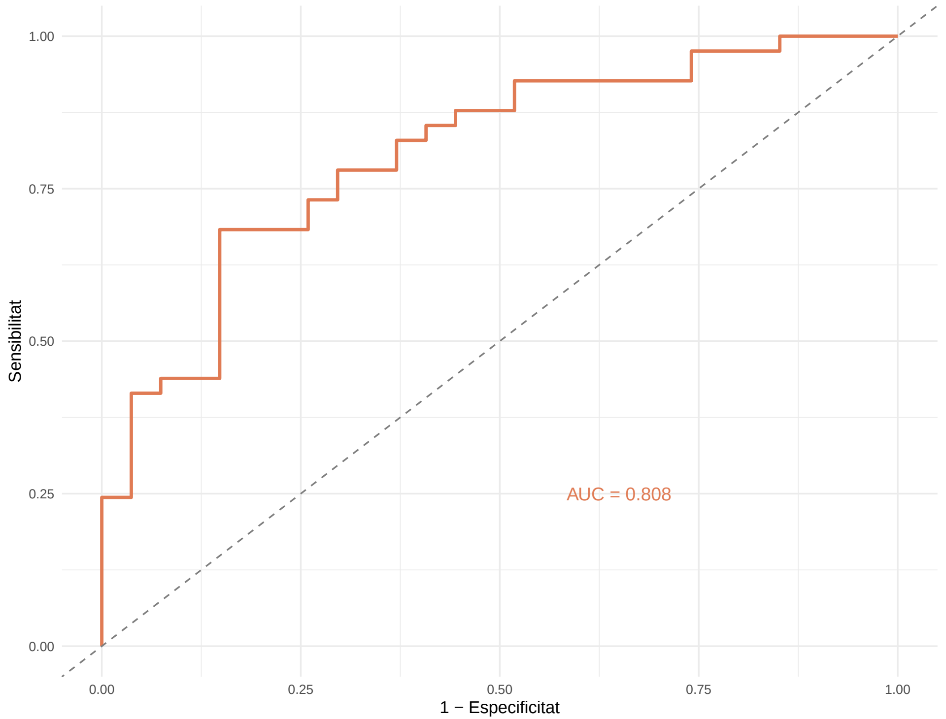
Corba ROC — RF-B
